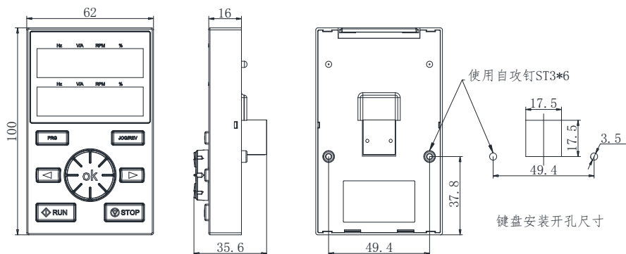
AC10 系列外引键盘尺寸
