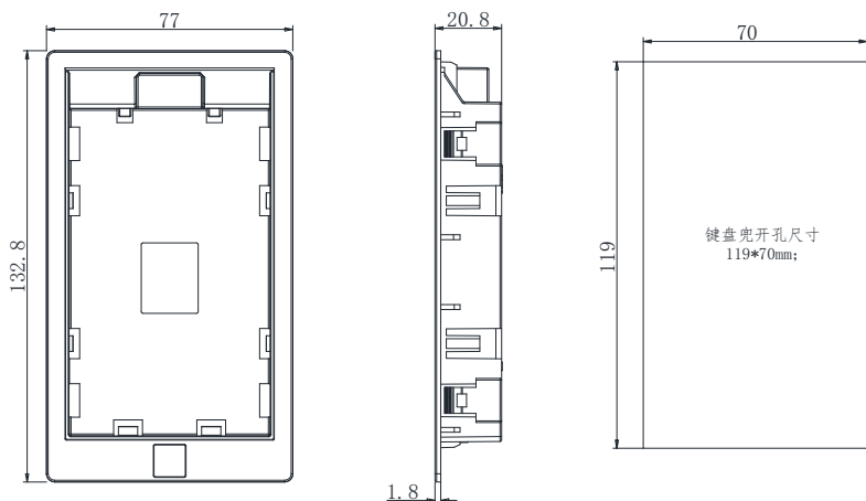
AC10 系列外引键盘兜外形及开孔尺寸图
