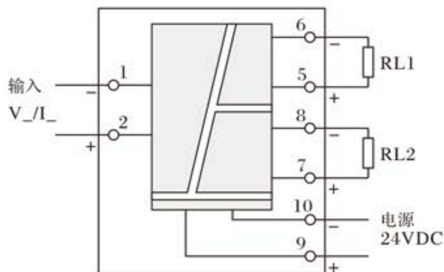
ABG...T 一入两出接线端子示意
