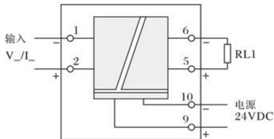
ABG...T 一入一出接线端子示意
