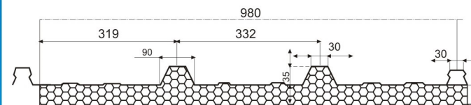
屋面组装
