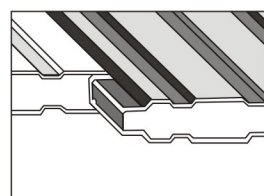
企口安装
