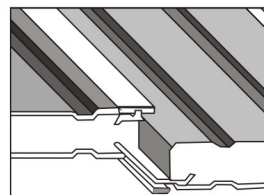
平板安装
