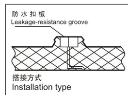
屋面组装
