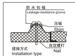
瓦楞组装
